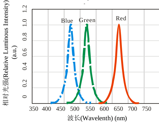
光谱分布特性曲线 Relative Spectral Distribution
