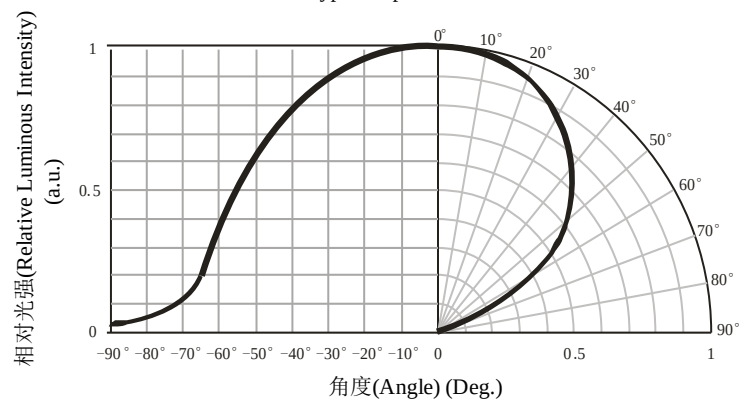
光强分布特性曲线 Typical Spatial Distribution
